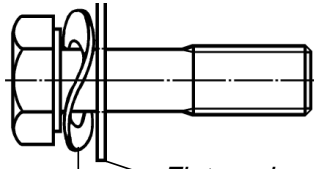
Flat washer B 5,5 DIN 6902 Curved spring washer 5,5 DIN 6904
